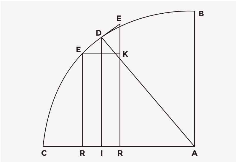
FIGURA 4: EL TRIÁNGULO CARACTERÍSTICO SEGÚN PASCAL. 18
