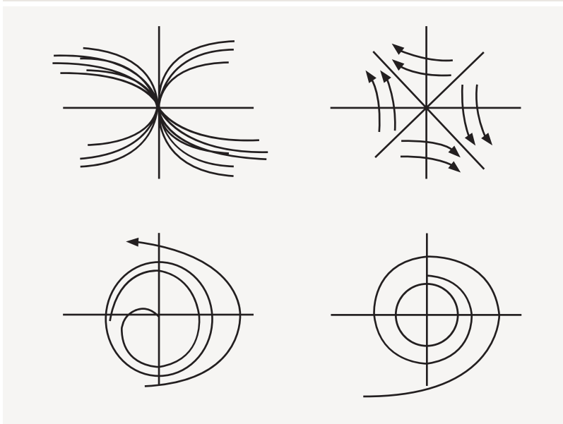
FIGURA 8: LOS PUNTOS SINGULARES DE POINCARÉ: NUDO, CUELLO, FOCO, CENTRO.
