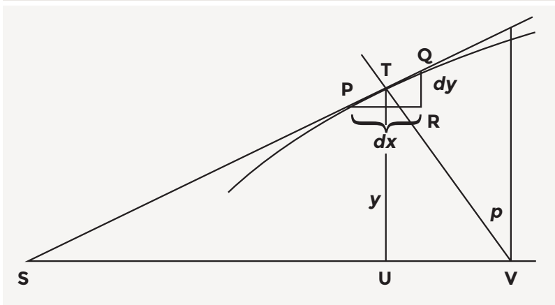
FIGURA 5: EL TRIÁNGULO CARACTERÍSTICO SEGÚN LEIBNIZ.
