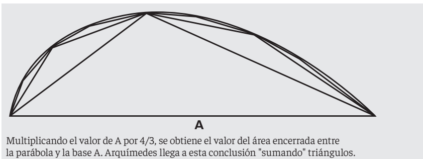
Figura 2: el cálculo de la superficie de la parábola por Arquímedes. 5
