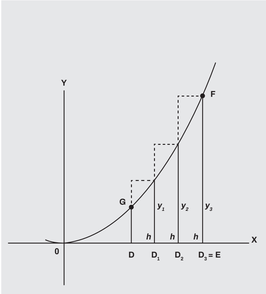
Figura 7: integral de la curva definida entre los puntos G y F, como suma de los rectángulos de base infinitamente delgada h y alturas variables y . 55
