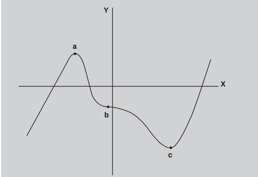
Figura 9: singularidades "ordinarias": máximo a, punto de inflexión b, mínimo c.
