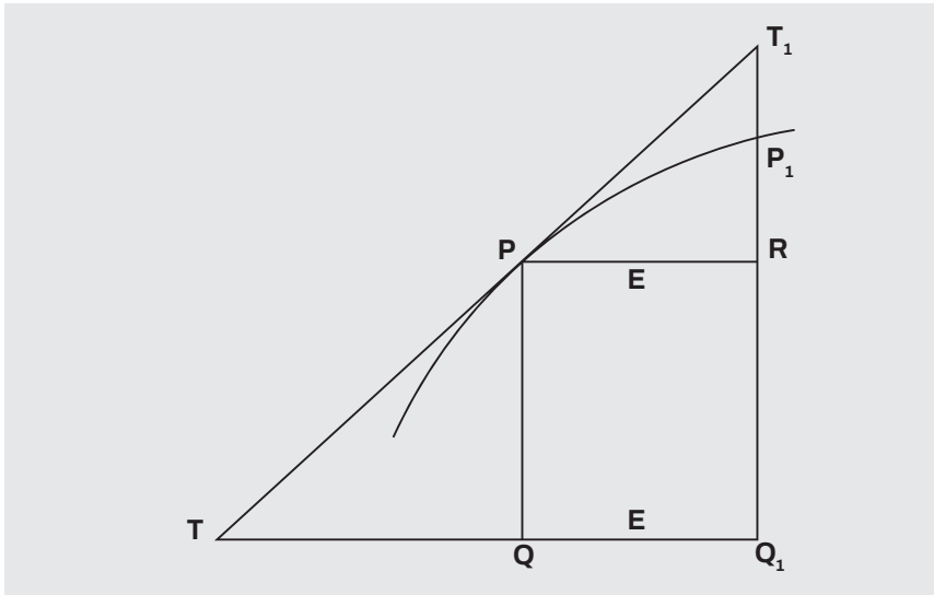
Figura 3: el método de las tangentes de Fermat. 15
