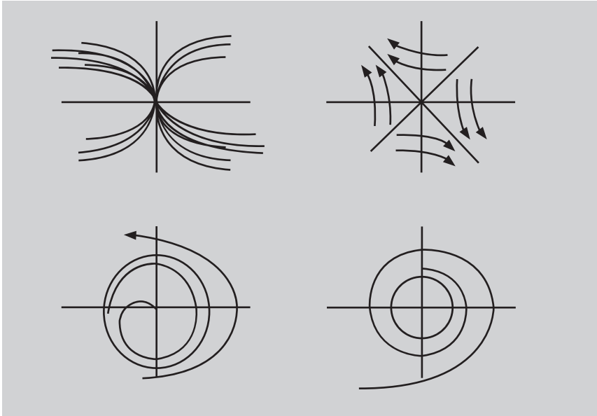
Figura 8: los puntos singulares de Poincaré: nudo, cuello, foco, centro.
