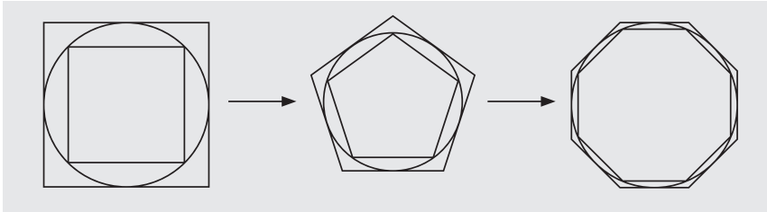
Figura 1: representación del método exhaustivo.
