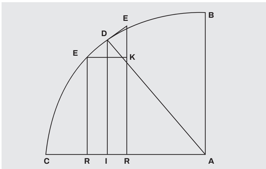
Figura 4: el triángulo característico según Pascal. 18
