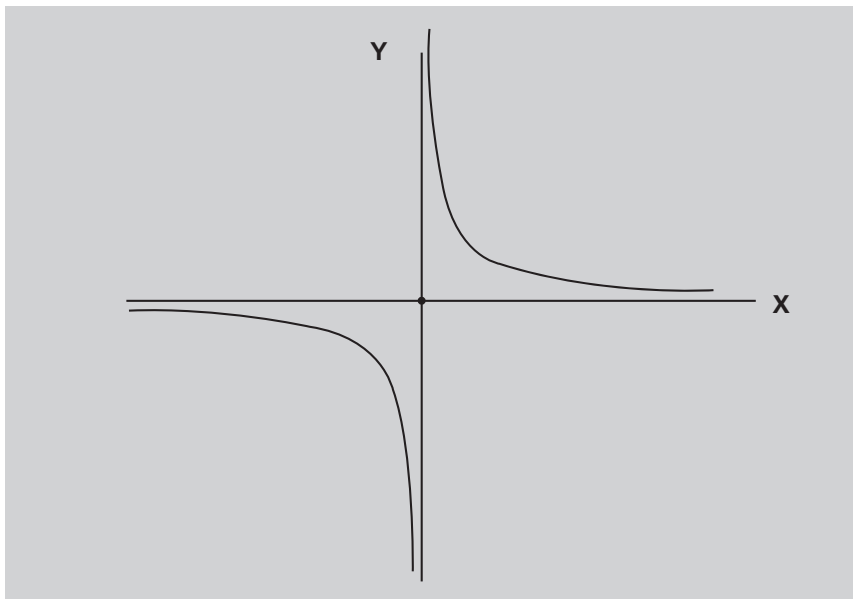
Figura 10: singularidad "notable" correspondiente a la función f(x)=\frac{1}{x} , con polo en x=0 .
