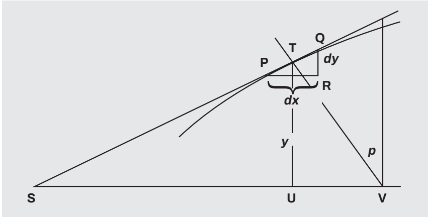
Figura 5: el triángulo característico según Leibniz.
